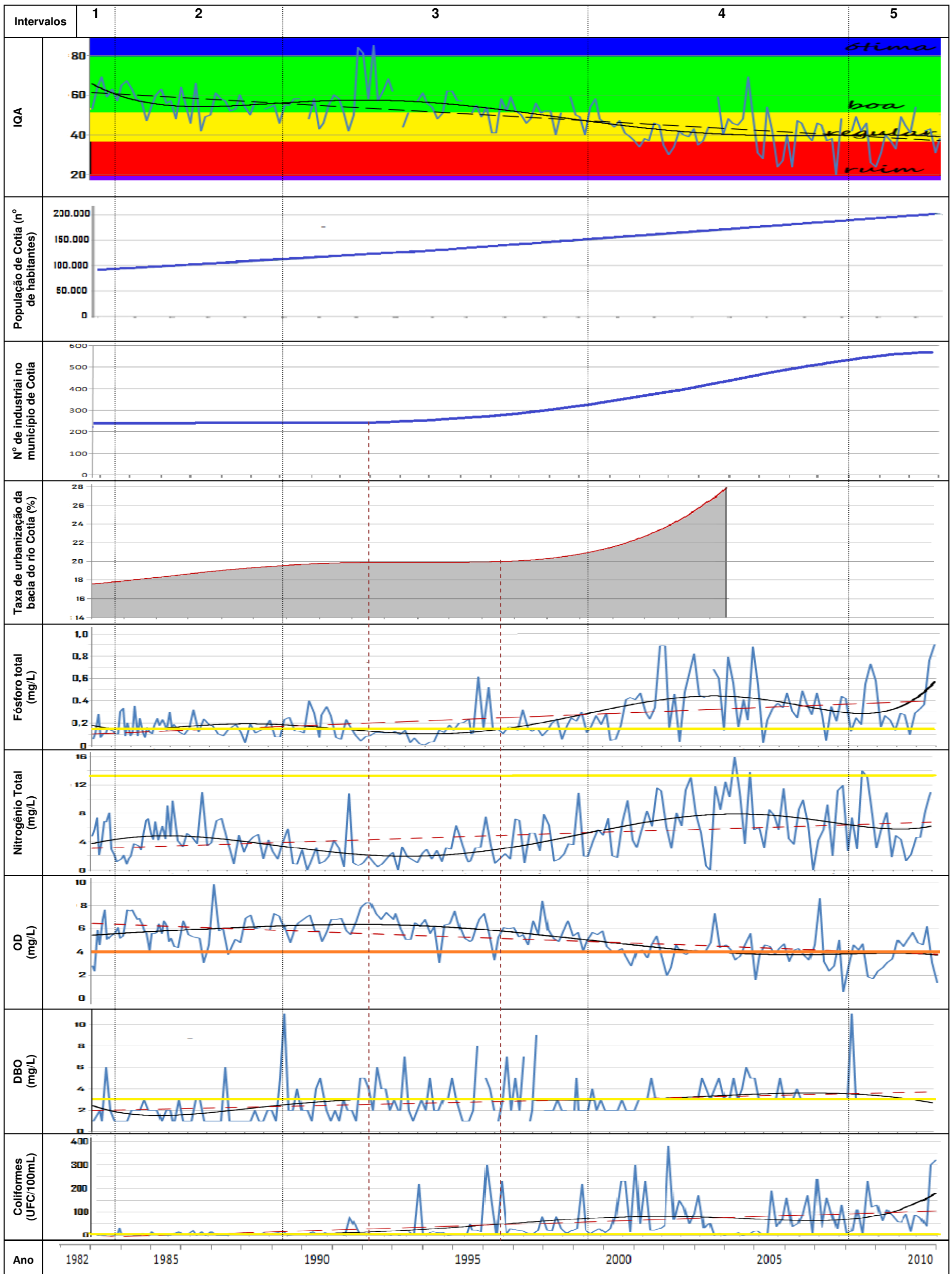
Gráfico 16 – Ponto de monitoramento Cotia Baixo: Comparação da evolução IQA, da população do município de Cotia (nº de habitantes), número de indústrias e taxa de urbanização à montante do ponto Cotia Baixo e respectivos parâmetros impactantes ao IQA (1982 a 2010). Fonte: CETESB (1989,....,2011), BRASIL (2005). Dados trabalhados pelo autor.
