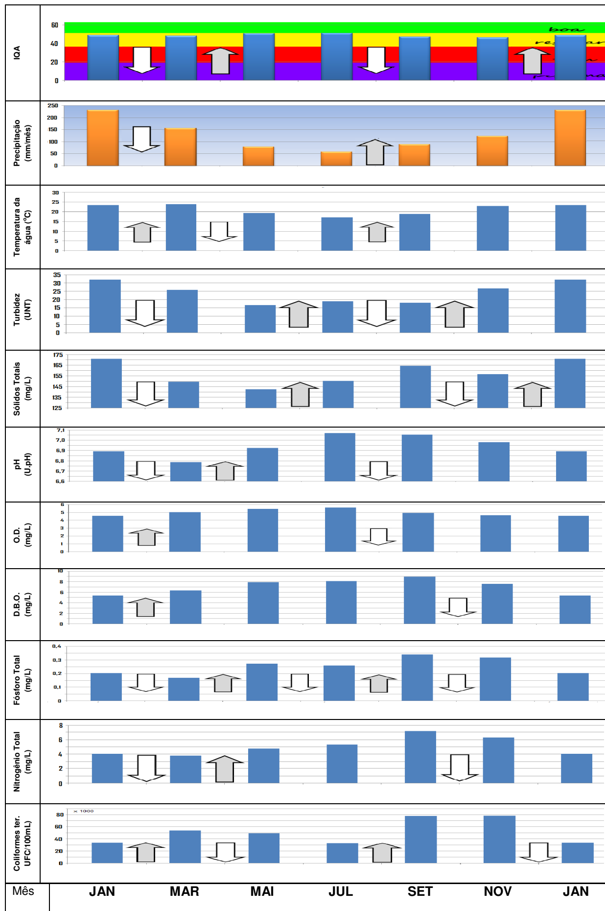
Gráfico 19 - Cotia Baixo: tendências sazonais dos parâmetros do IQA, inclusive IQA, com base nas médias mensais (1982 a 2010: meses ímpares). Fonte: CETESB (1983, ..., 2011).
